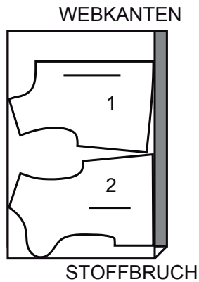
WEBKANTEN
